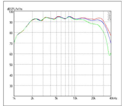
SPL VERTIKAL 0° - 5° - 15°
